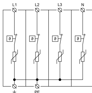
Vnútrotná schéma zapojenia
