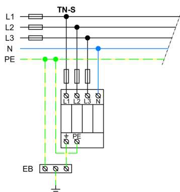
Aplikačná schéma zapojenia (inštalácia)
